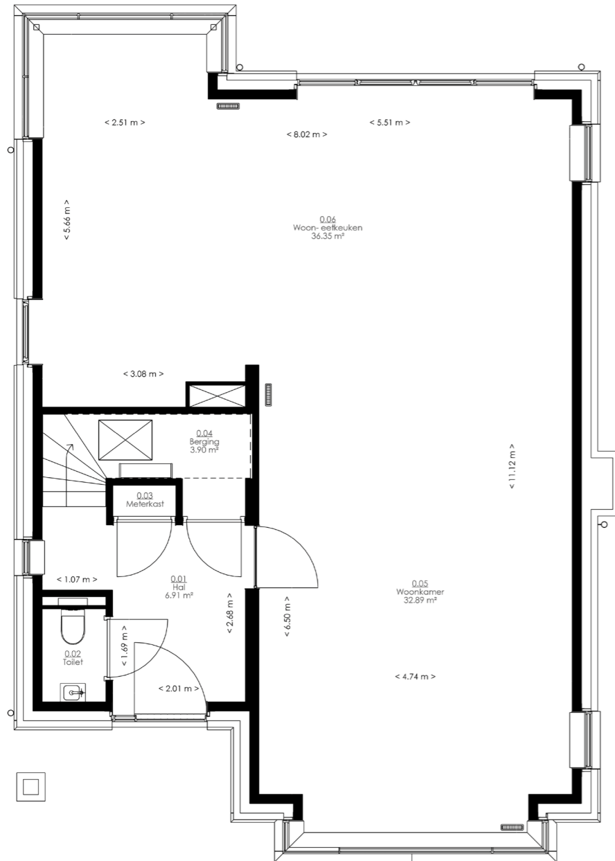
BEGANE GROND
